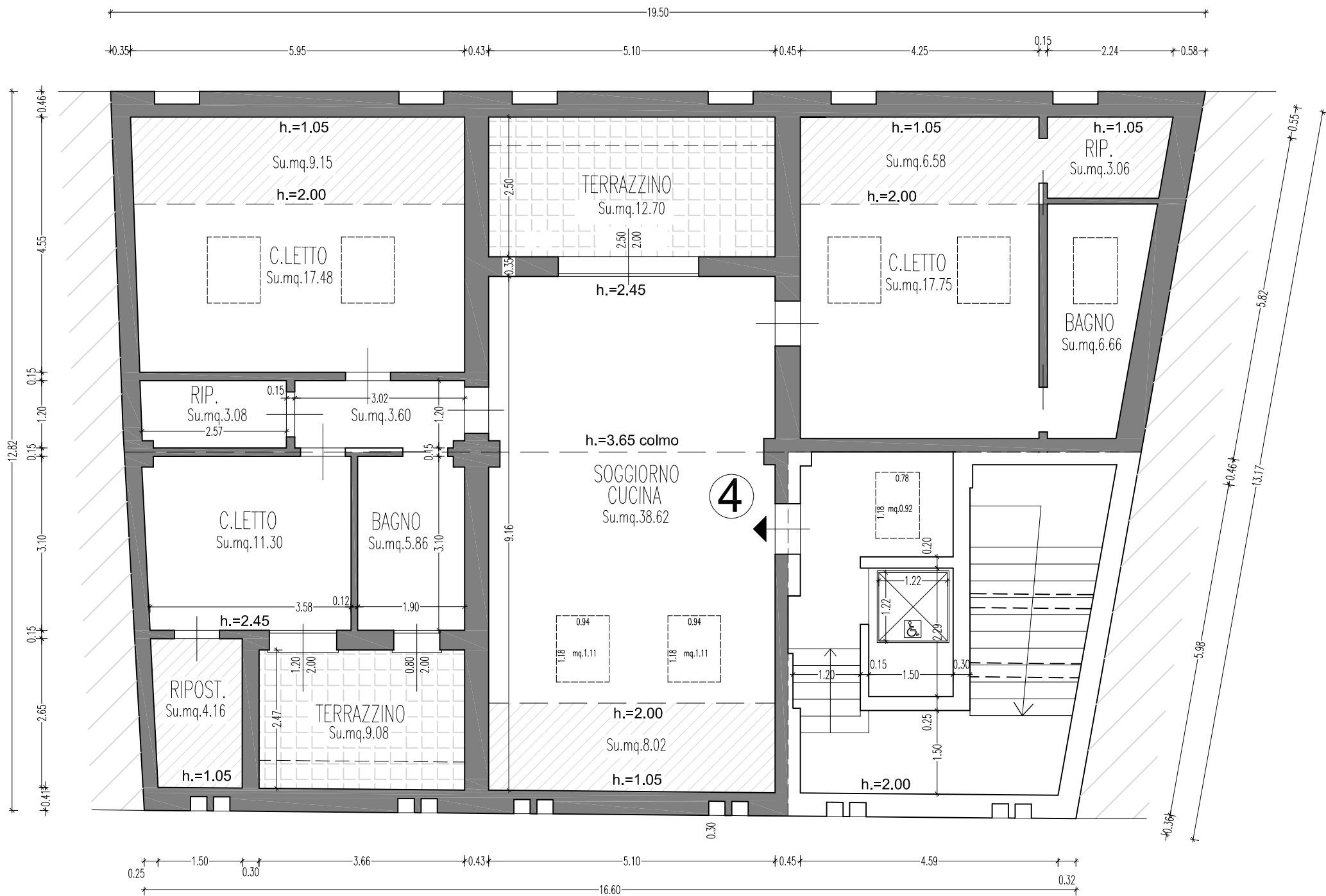
Piano Sottotetto
